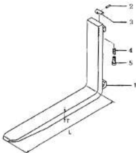
货叉总成 Fork Ass'y
